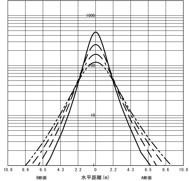
○直射水平面照度 (全光束: 3080 × 1 = 3080lm/台) 照度 (lx) — H1.50m --- H2.00m - - - H2.50m - · - · H3.00m (保守率: 1.00)
