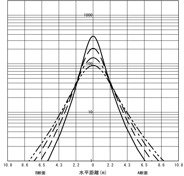
○直射水平面照度 (全光束: 2450 × 1 = 2450lm/台) 照度 (lx) — H1.50m --- H2.00m - - - H2.50m - · - · H3.00m (保守率: 1.00)
