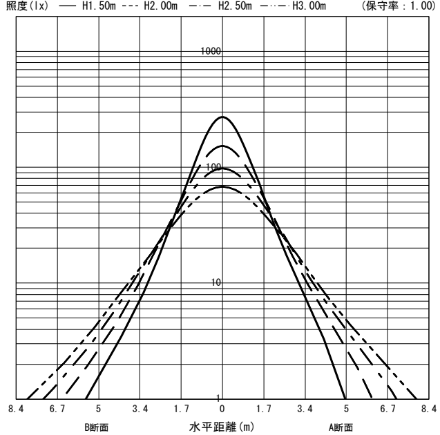
○直射水平面照度 (全光束: 1760 × 1 = 1760lm/台)
