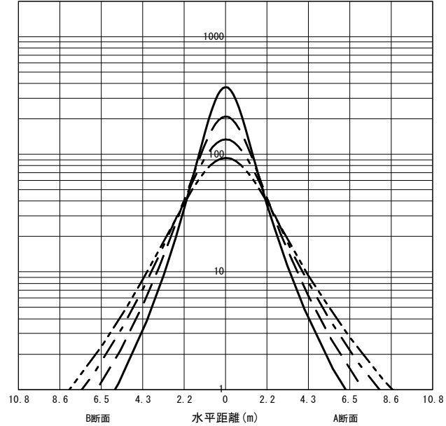
○直射水平面照度 (全光束: 2420 × 1 = 2420lm/台) 照度 (lx) — H1.50m --- H2.00m - - - H2.50m - · - · H3.00m (保守率: 1.00)
