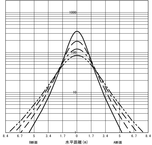
○直射水平面照度 (全光束 : 2130 × 1 = 2130lm/台) 照度 (lx) — H1.50m --- H2.00m - - - H2.50m - · - · H3.00m (保守率 : 1.00)
