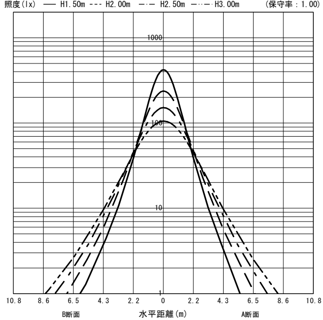
○直射水平面照度 (全光束: 2640 × 1 = 2640lm/台)
