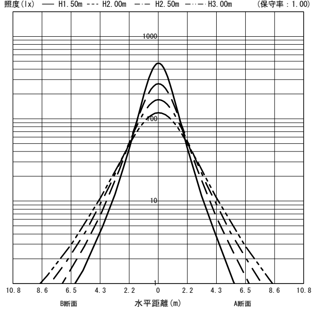
○直射水平面照度 (全光束 : 2970 × 1 = 2970lm/台)
