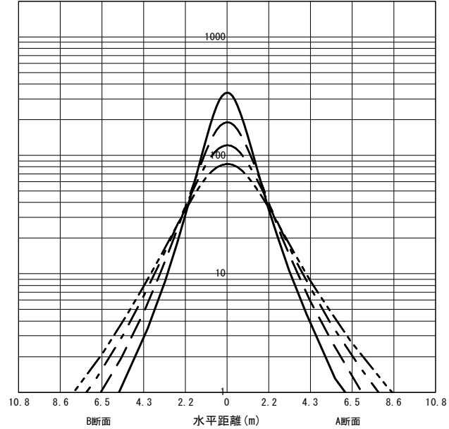
○直射水平面照度 (全光束 : 2230 × 1 = 2230lm/台)
