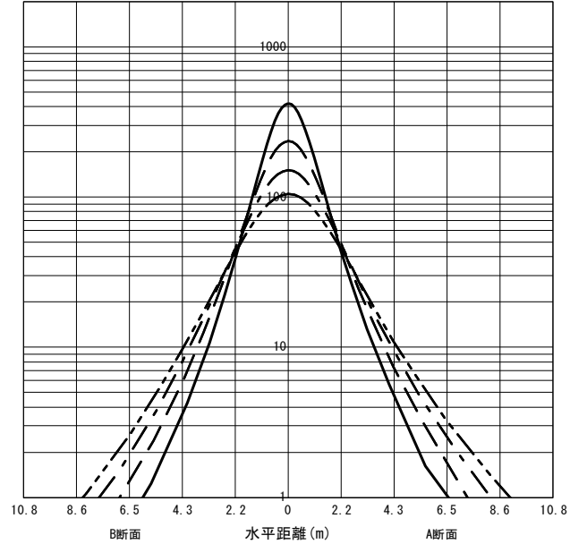
○直射水平面照度 (全光束: 2760 × 1 = 2760lm/台) 照度 (lx) — H1.50m --- H2.00m - - - H2.50m - · - · H3.00m (保守率: 1.00)
