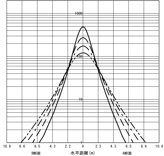
○直射水平面照度 (全光束: 3100 × 1 = 3100lm/台) 照度 (lx) — H1.50m --- H2.00m - - - H2.50m - · - · H3.00m (保守率: 1.00)
