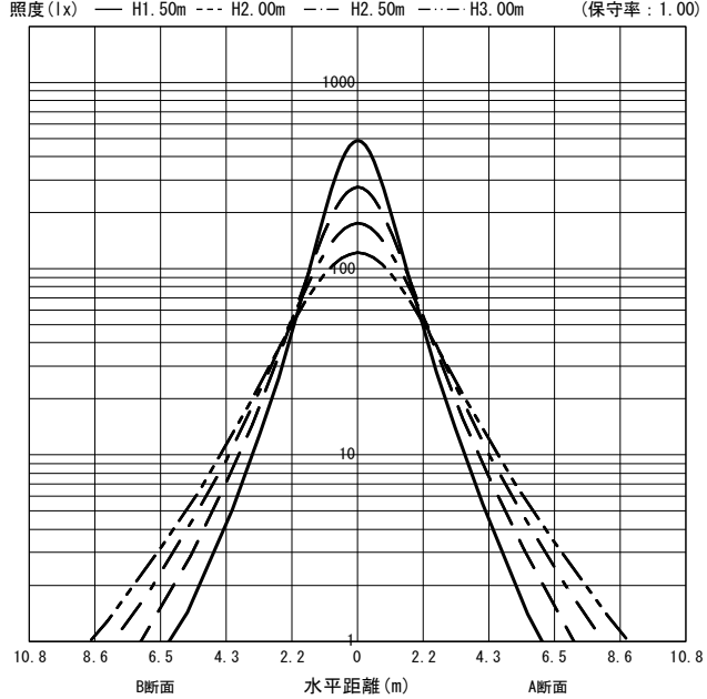
○直射水平面照度 (全光束: 3100 × 1 = 3100lm/台)
