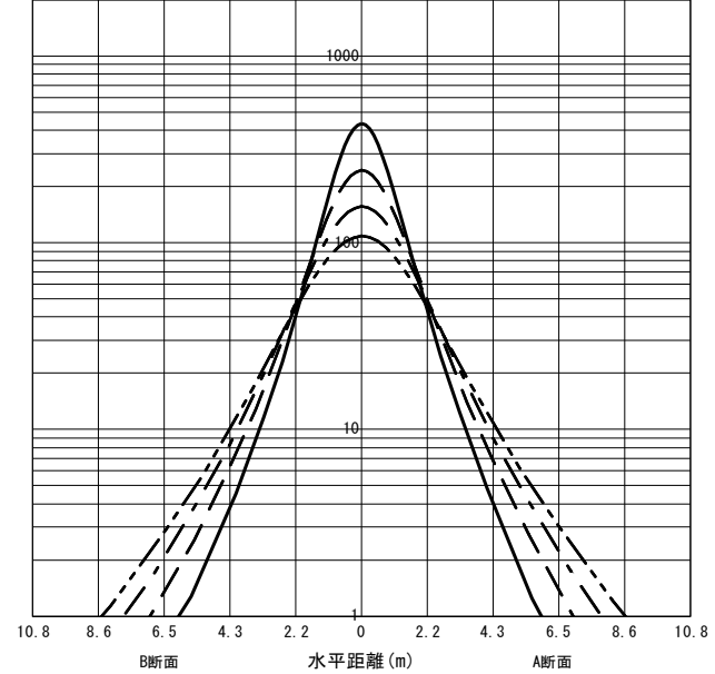
○直射水平面照度 (全光束: 2760 × 1 = 2760lm/台)
