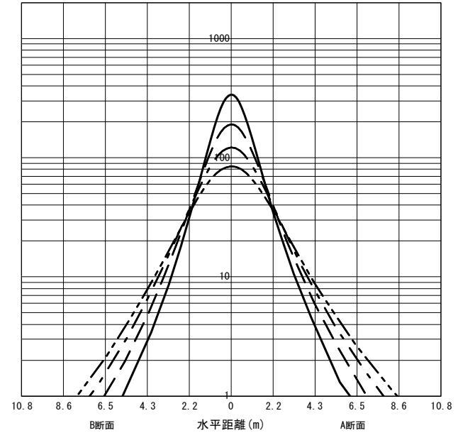
○直射水平面照度 (全光束 : 2230 × 1 = 2230lm/台) 照度 (lx) — H1.50m --- H2.00m - - - H2.50m - · - · - H3.00m (保守率 : 1.00)
