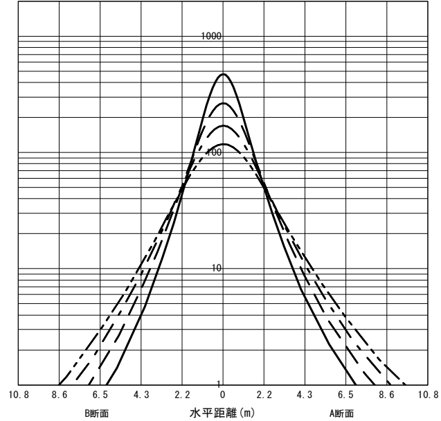
○直射水平面照度 (全光束: 3130 × 1 = 3130lm/台) 照度 (lx) — H1.50m --- H2.00m - - - H2.50m - · - · H3.00m (保守率: 1.00)
