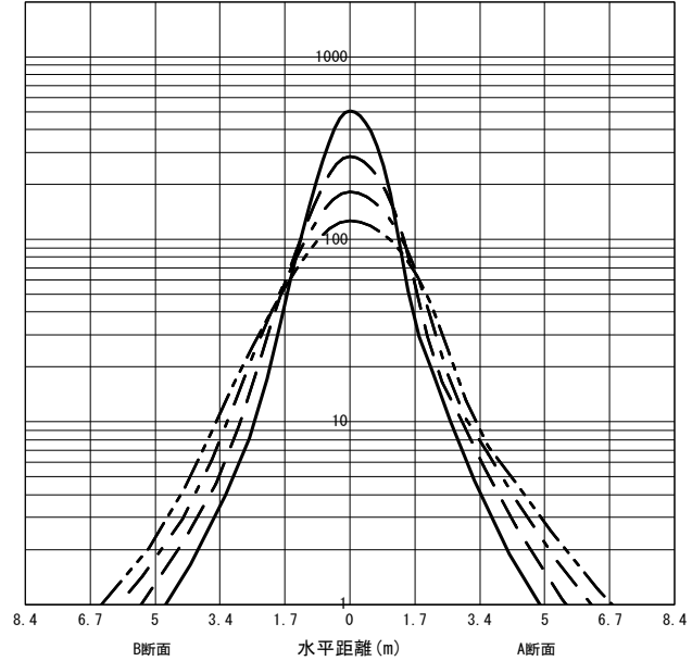
○直射水平面照度 (全光束: 1960 × 1 = 1960lm/台) 照度 (lx) — H1.50m --- H2.00m - - - H2.50m - · - · H3.00m (保守率: 1.00)
