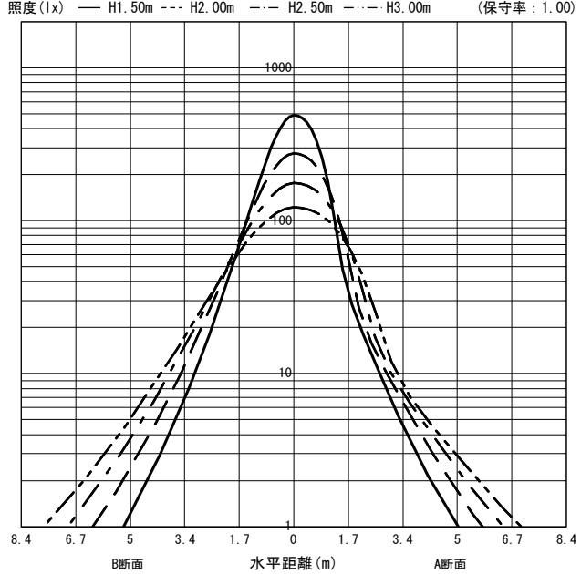
○直射水平面照度 (全光束: 2270 × 1 = 2270lm/台)
