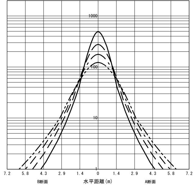
○直射水平面照度 (全光束: 1520 × 1 = 1520lm/台) 照度 (lx) — H1.50m --- H2.00m - - - H2.50m - · - · H3.00m (保守率: 1.00)
