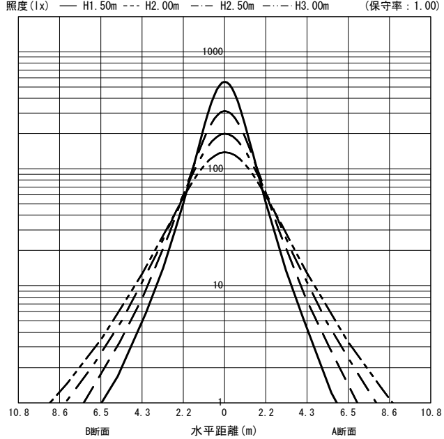
○直射水平面照度 (全光束: 3470 × 1 = 3470lm/台)
