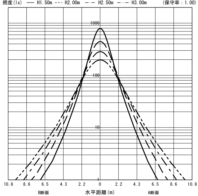
○直射水平面照度 (全光束: 5030 × 1 = 5030lm/台)
