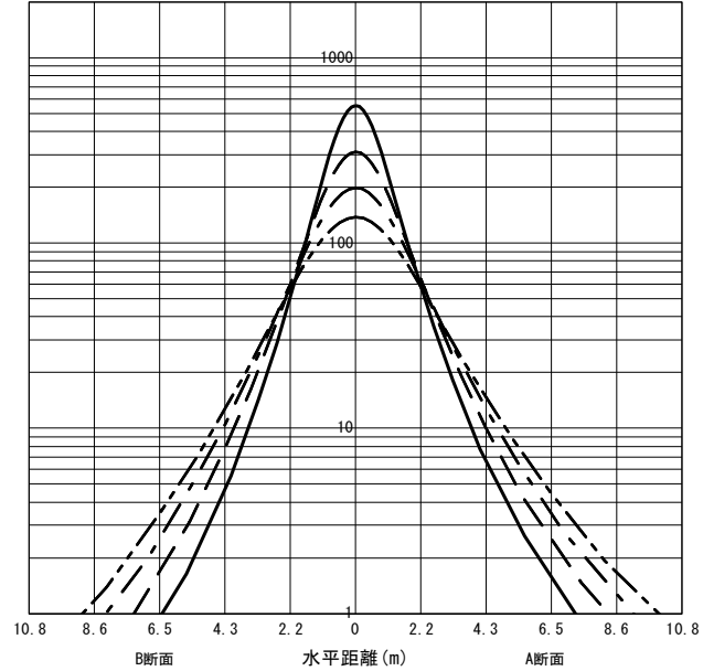
○直射水平面照度 (全光束: 3660 × 1 = 3660lm/台) 照度 (lx) — H1.50m --- H2.00m - - - H2.50m - · - · H3.00m (保守率: 1.00)
