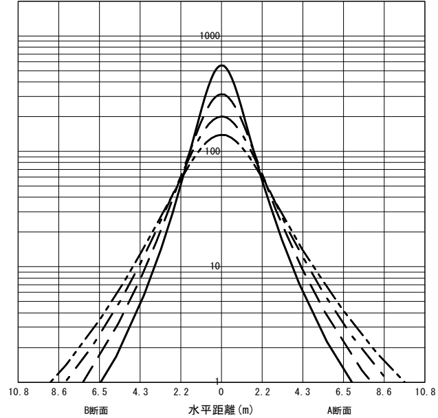
○直射水平面照度 (全光束: 3620 × 1 = 3620lm/台) 照度 (lx) — H1.50m --- H2.00m - - - H2.50m - · - · H3.00m (保守率: 1.00)
