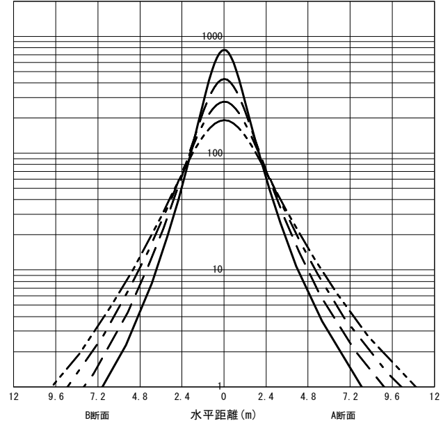
○直射水平面照度 (全光束: 5090 × 1 = 5090lm/台) 照度 (lx) — H1.50m --- H2.00m - - - H2.50m - · - · H3.00m (保守率: 1.00)
