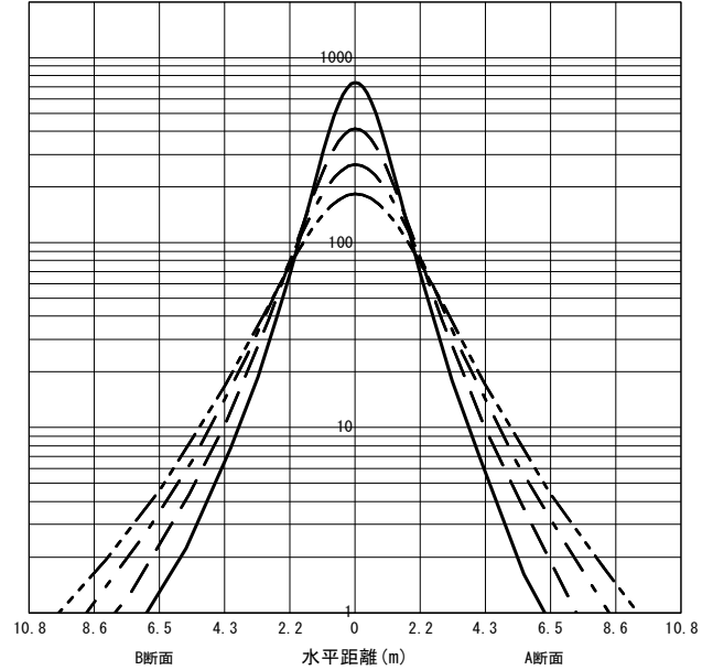
○直射水平面照度 (全光束：4600 × 1 = 4600lm/台) 照度 (lx) — H1.50m --- H2.00m - - - H2.50m - · - H3.00m (保守率：1.00)
