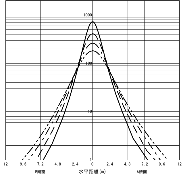
○直射水平面照度 (全光束: 4800 × 1 = 4800lm/台) 照度 (lx) — H1.50m --- H2.00m - - - H2.50m - · - · H3.00m (保守率: 1.00)
