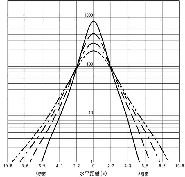
○直射水平面照度 (全光束: 4850 × 1 = 4850lm/台) 照度 (lx) — H1.50m --- H2.00m - - - H2.50m - · - · H3.00m (保守率: 1.00)
