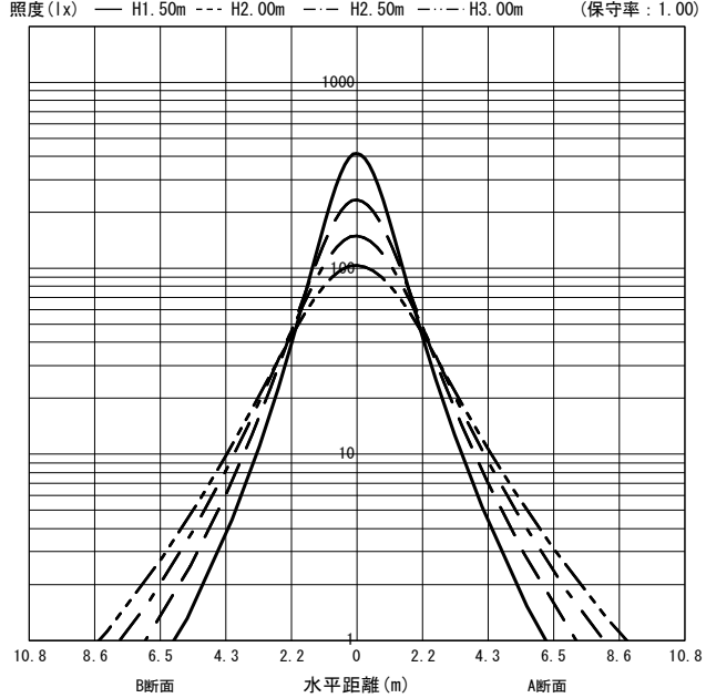
○直射水平面照度 (全光束: 2730 × 1 = 2730lm/台)
