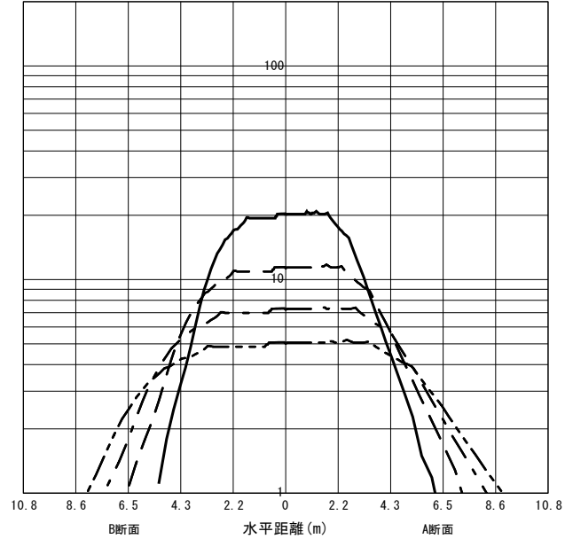
○直射水平面照度 (全光束 : 841 × 1 = 841lm/台) 照度 (lx) — H1.50m --- H2.00m - - - H2.50m - · - · H3.00m (保守率 : 1.00)
