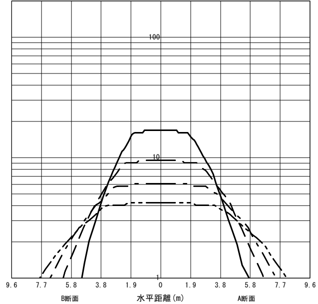
○直射水平面照度 (全光束 : 667 × 1 = 667lm/台) 照度 (lx) — H1.50m --- H2.00m - - - H2.50m - · - · H3.00m (保守率 : 1.00)
