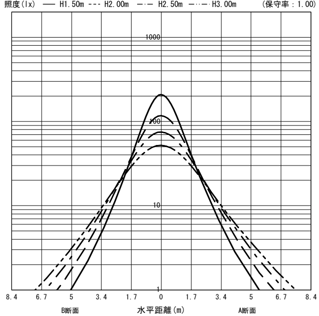
○直射水平面照度 (全光束: 1390 × 1 = 1390lm/台)
