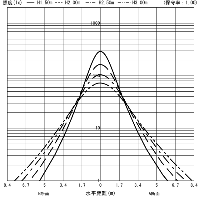
○直射水平面照度 (全光束: 1940 × 1 = 1940lm/台)
