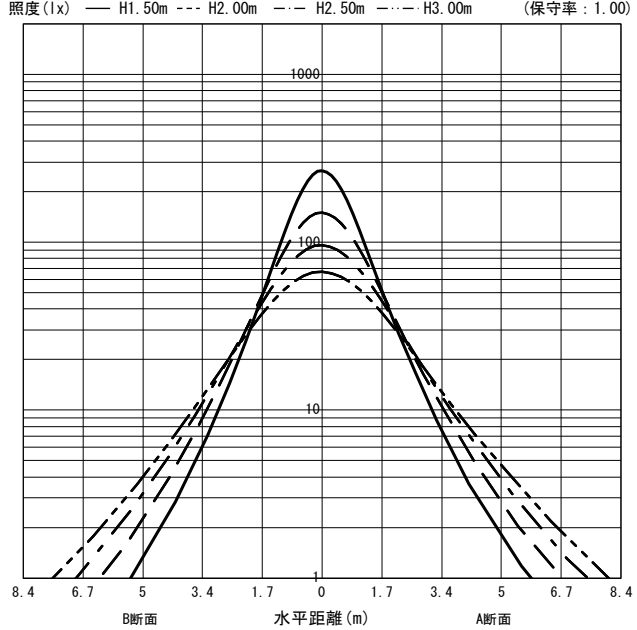
○直射水平面照度 (全光束: 1780 × 1 = 1780lm/台)
