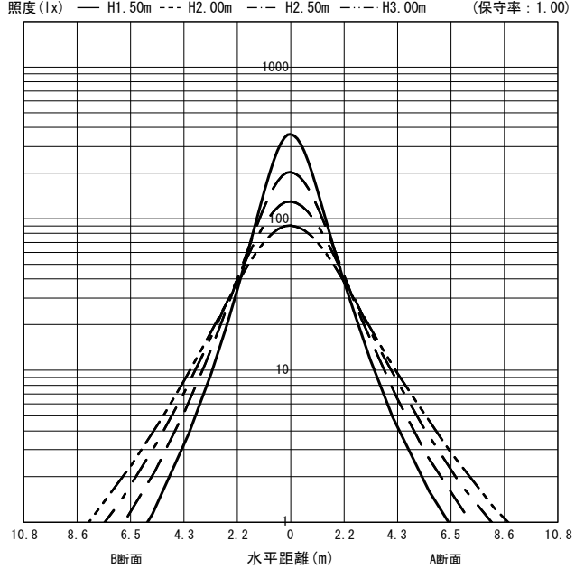
○直射水平面照度 (全光束: 2410 × 1 = 2410lm/台)
