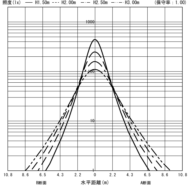
○直射水平面照度 (全光束: 2950 × 1 = 2950lm/台)
