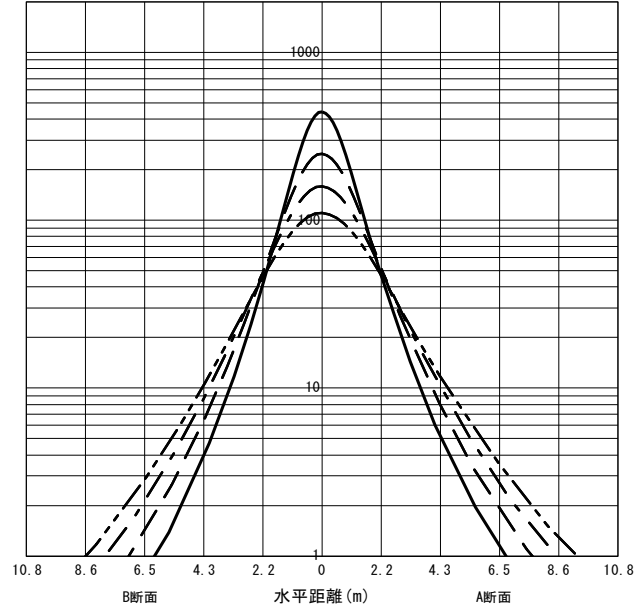
○直射水平面照度 (全光束: 2950 × 1 = 2950lm/台) 照度 (lx) — H1.50m --- H2.00m - - - H2.50m - · - · H3.00m (保守率: 1.00)
