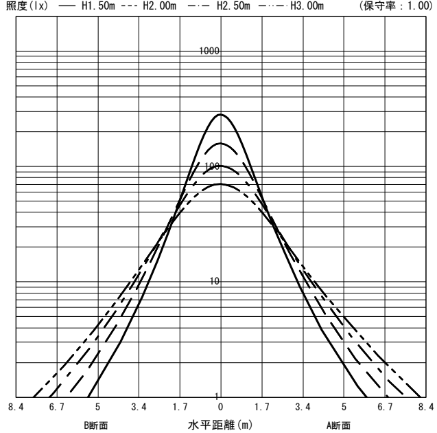
○直射水平面照度 (全光束: 1880 × 1 = 1880lm/台)
