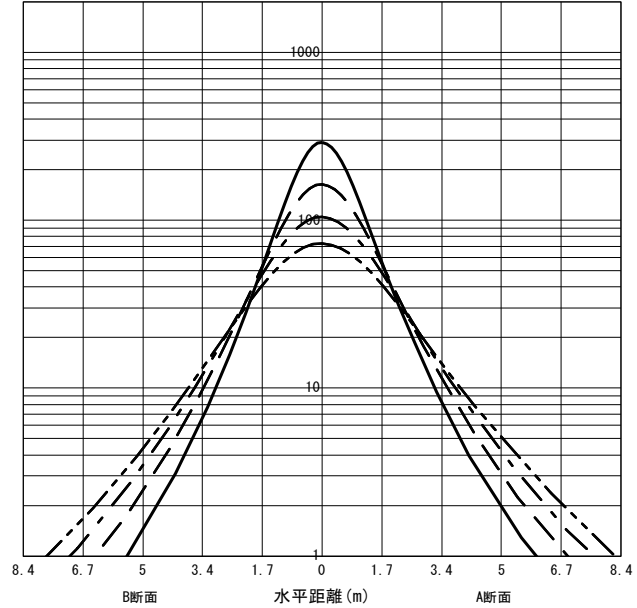
○直射水平面照度 (全光束: 1940 × 1 = 1940lm/台) 照度 (lx) — H1.50m --- H2.00m - - - H2.50m - · - · H3.00m (保守率: 1.00)
