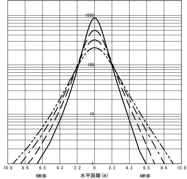
○直射水平面照度 (全光束: 5830 × 1 = 5830lm/台) 照度 (lx) — H1.50m --- H2.00m - - - H2.50m - · - · H3.00m (保守率: 1.00)
