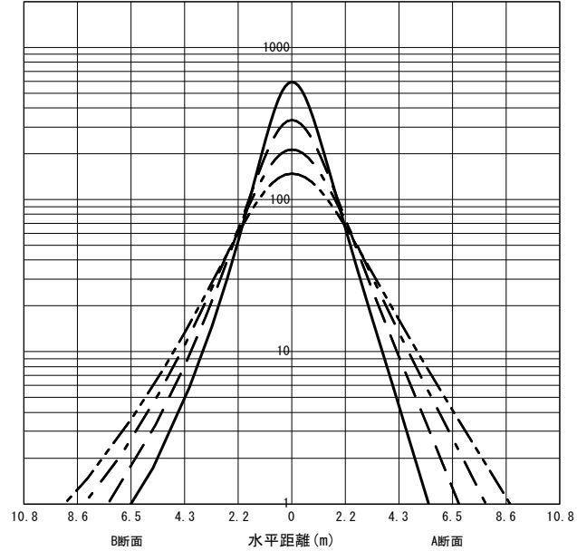
○直射水平面照度 (全光束: 3850 × 1 = 3850lm/台) 照度 (lx) — H1.50m --- H2.00m - - - H2.50m - · - · H3.00m (保守率: 1.00)
