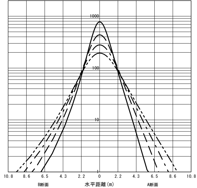
○直射水平面照度 (全光束: 5050 × 1 = 5050lm/台) 照度 (lx) — H1.50m --- H2.00m - - - H2.50m - · - · H3.00m (保守率: 1.00)
