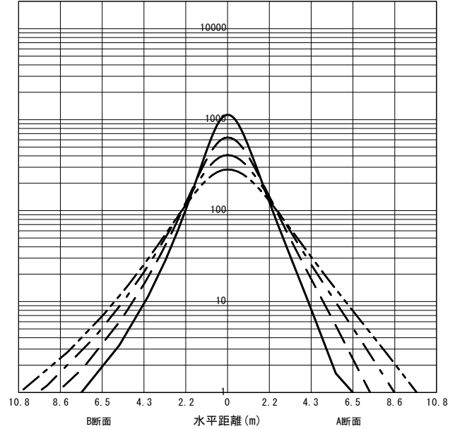
○直射水平面照度 (全光束: 7350 × 1 = 7350lm/台) 照度 (lx) — H1.50m --- H2.00m - - - H2.50m - · - · H3.00m (保守率: 1.00)
