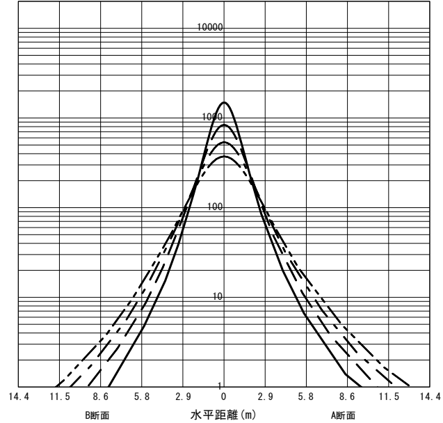
○直射水平面照度 (全光束: 9780 × 1 = 9780lm/台) 照度 (lx) — H1.50m --- H2.00m - - - H2.50m - · - · H3.00m (保守率: 1.00)
