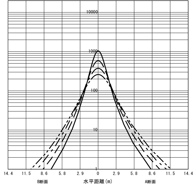
○直射水平面照度 (全光束 : 6850 × 1 = 6850lm/台) 照度 (lx) — H1.50m --- H2.00m - - - H2.50m - · - · H3.00m (保守率 : 1.00)
