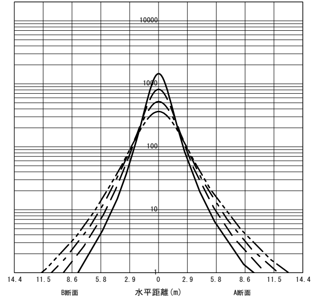
○直射水平面照度 (全光束: 9540 × 1 = 9540lm/台) 照度 (lx) — H1.50m --- H2.00m - - - H2.50m - · - · H3.00m (保守率: 1.00)
