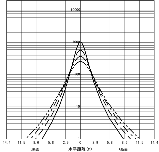
○直射水平面照度 (全光束: 6700 × 1 = 6700lm/台) 照度 (lx) — H1.50m --- H2.00m - - - H2.50m - · - · H3.00m (保守率: 1.00)
