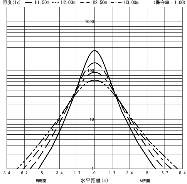
○直射水平面照度 (全光束: 1700 × 1 = 1700lm/台)
