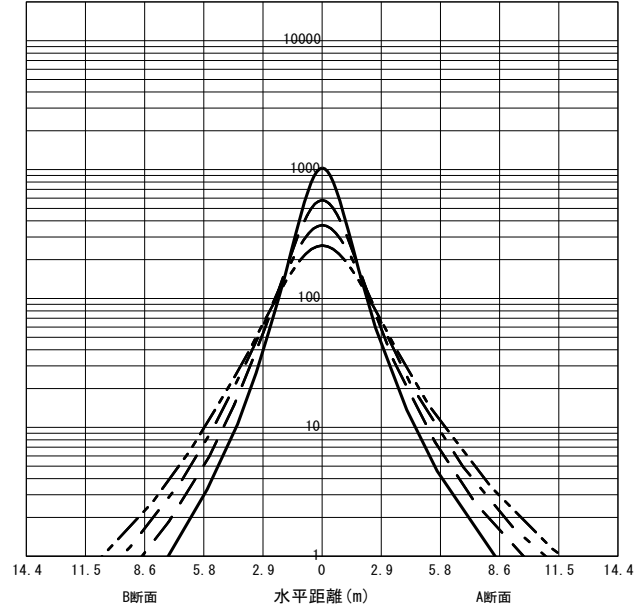
○直射水平面照度 (全光束: 6750 × 1 = 6750lm/台) 照度 (lx) — H1.50m --- H2.00m - - - H2.50m - · - · H3.00m (保守率: 1.00)
