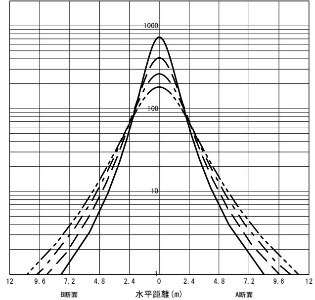
○直射水平面照度 (全光束: 5200 × 1 = 5200lm/台) 照度 (lx) — H1.50m --- H2.00m - - - H2.50m - · - · H3.00m (保守率: 1.00)
