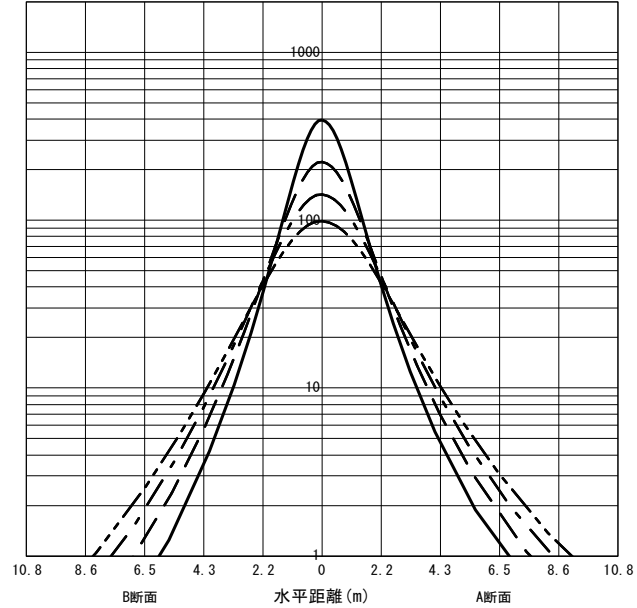
○直射水平面照度 (全光束: 2820 × 1 = 2820lm/台) 照度 (lx) — H1.50m --- H2.00m - - - H2.50m - · - · H3.00m (保守率: 1.00)
