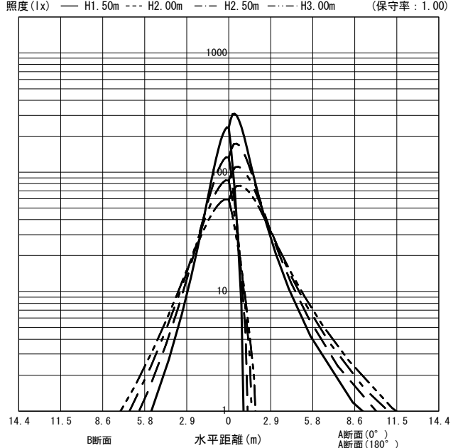
○直射水平面照度 (全光束: 2180 × 1 = 2180lm/台)
