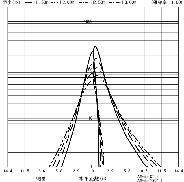
○直射水平面照度 (全光束: 2180 × 1 = 2180lm/台)
